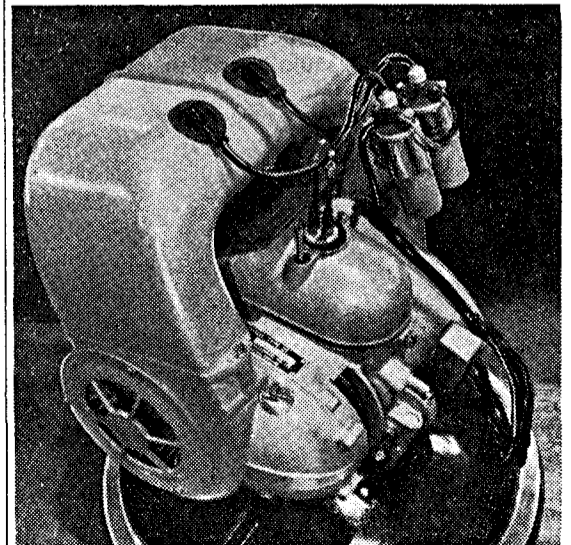
DER VILLIERS-ZWEITAKTER DES FRISKY Der luftgekühlte Zweizylinder-Zweitaktmotor wurde von Villiers speziell für Kleinstwagen entworfen und mit einem Viergang-Getriebe kombiniert. Die Leistung des 246-cm 3 -Motors beträgt 15 PS bei 5500 U/min.
